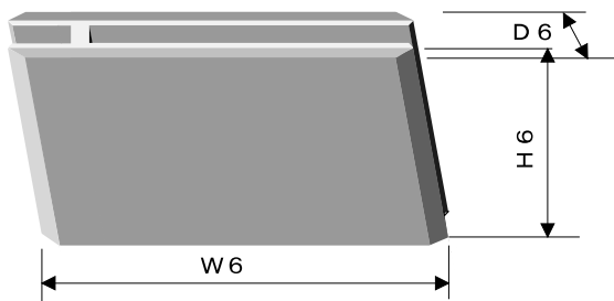
LKCP 6 (目地幅6mm用)
